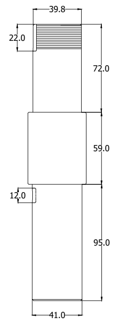
VISTA LATERAL
